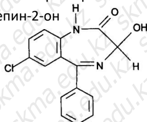
Nozepamum (Тазепам)
