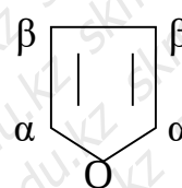
фуран
