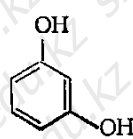
резорцин
