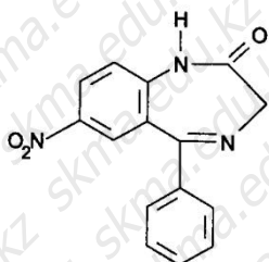
Nitrazepanum
