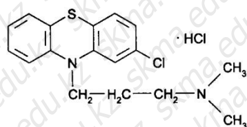
Аминазин – Aminazinum.
