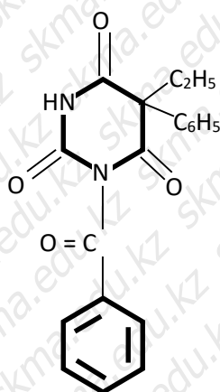
Бензонал – Benzonalum.
