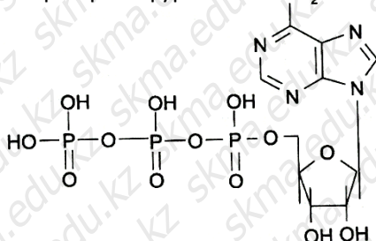
Acidum adenosintriphosphoricum
