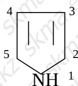
пиррол
