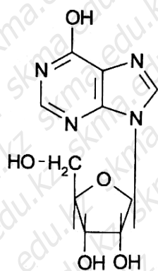
Riboxinum
