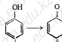
гидрохинон
